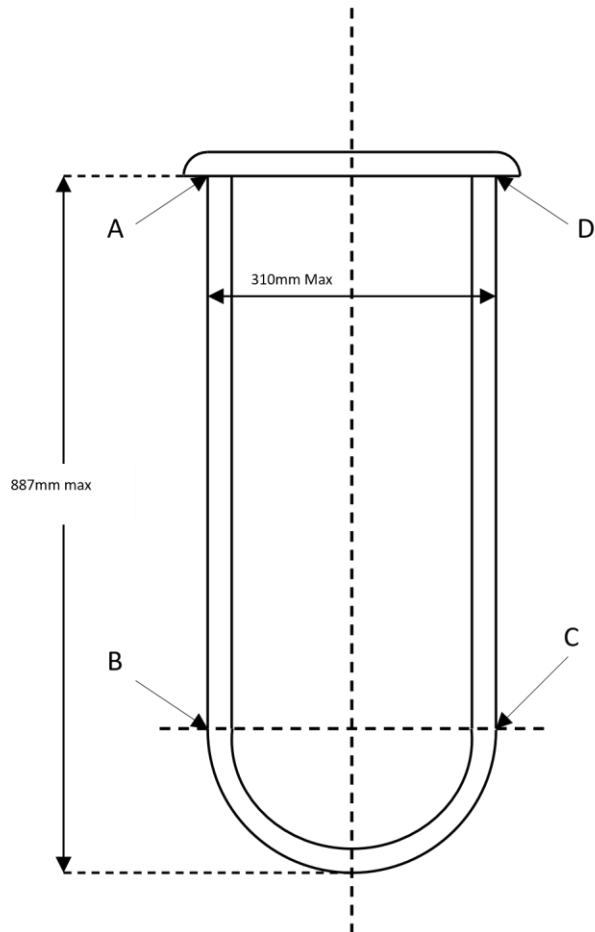
Daggerboard
